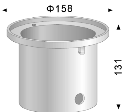
BOITIER D'ENCASTREMENT
